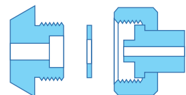
CGA 660 1.03" -14 带垫片
