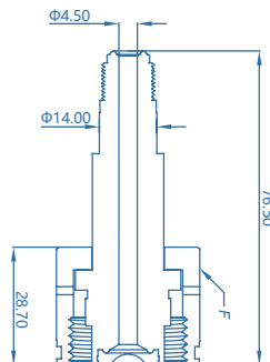
1/4" 密封件
