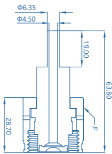
1/4" 焊接管
