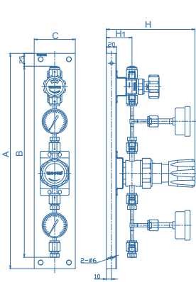
VUP-100TG (C型)
