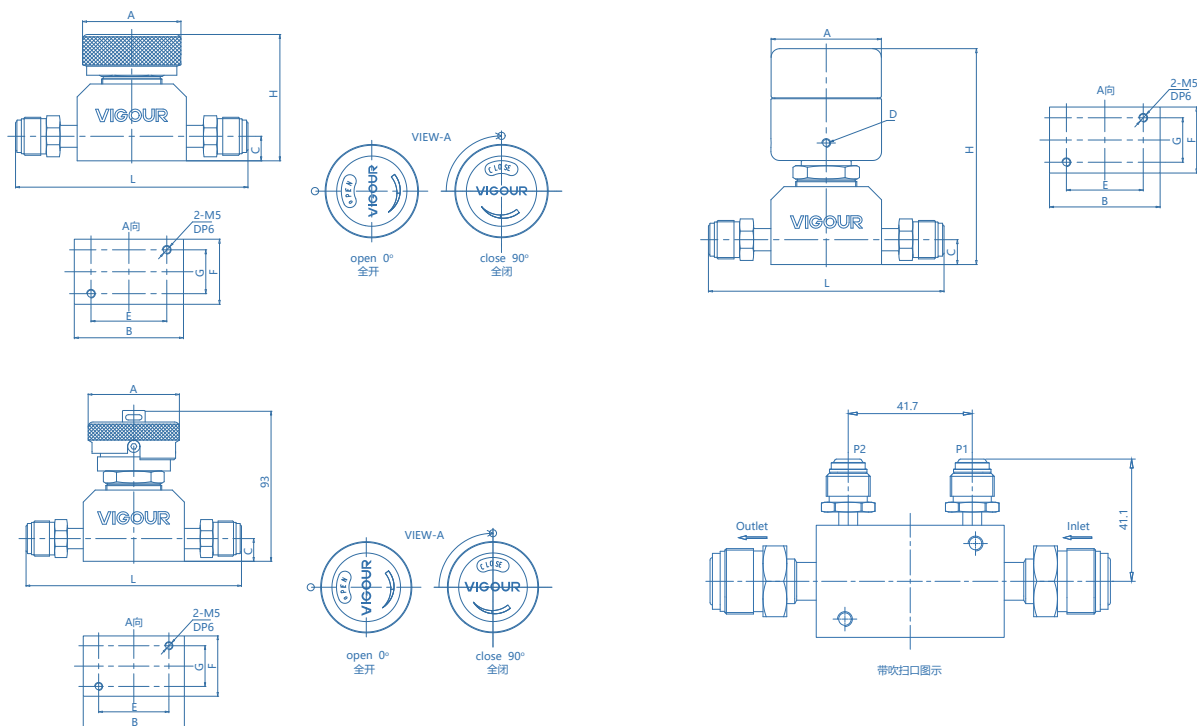
气动型 (常闭)
