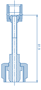
钢瓶接头转 1/4" VFS 内螺纹
