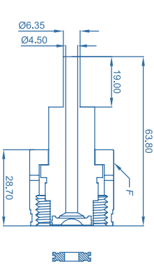
1/4" 焊接接管
