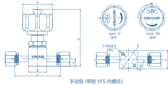
手动型 (带锁)
