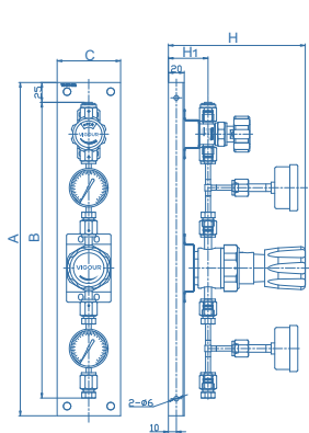
VUP-100TG (C 型)
