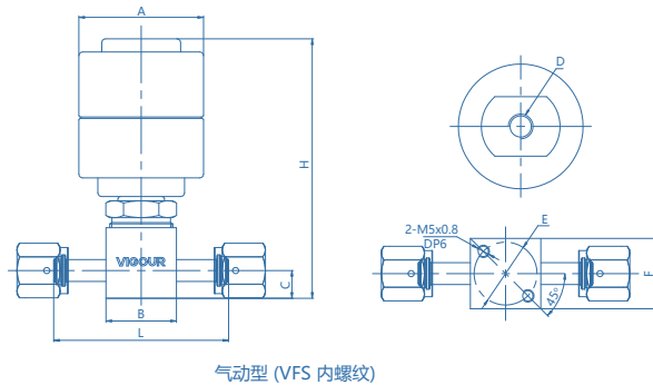
气动型 (常闭)
