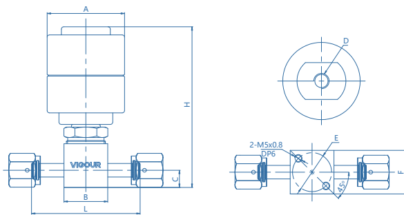
气动型 (常闭)
