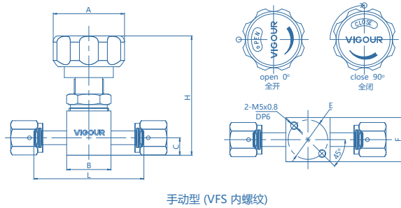
手动型
