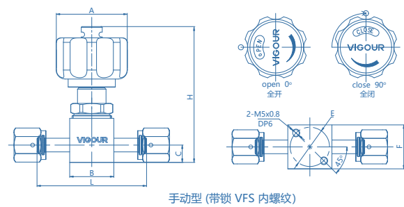
手动型 (带锁)
