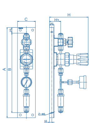
VUP-100TG (B 型)
